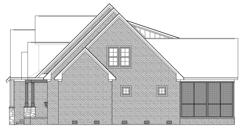
RIGHT ELEVATION
